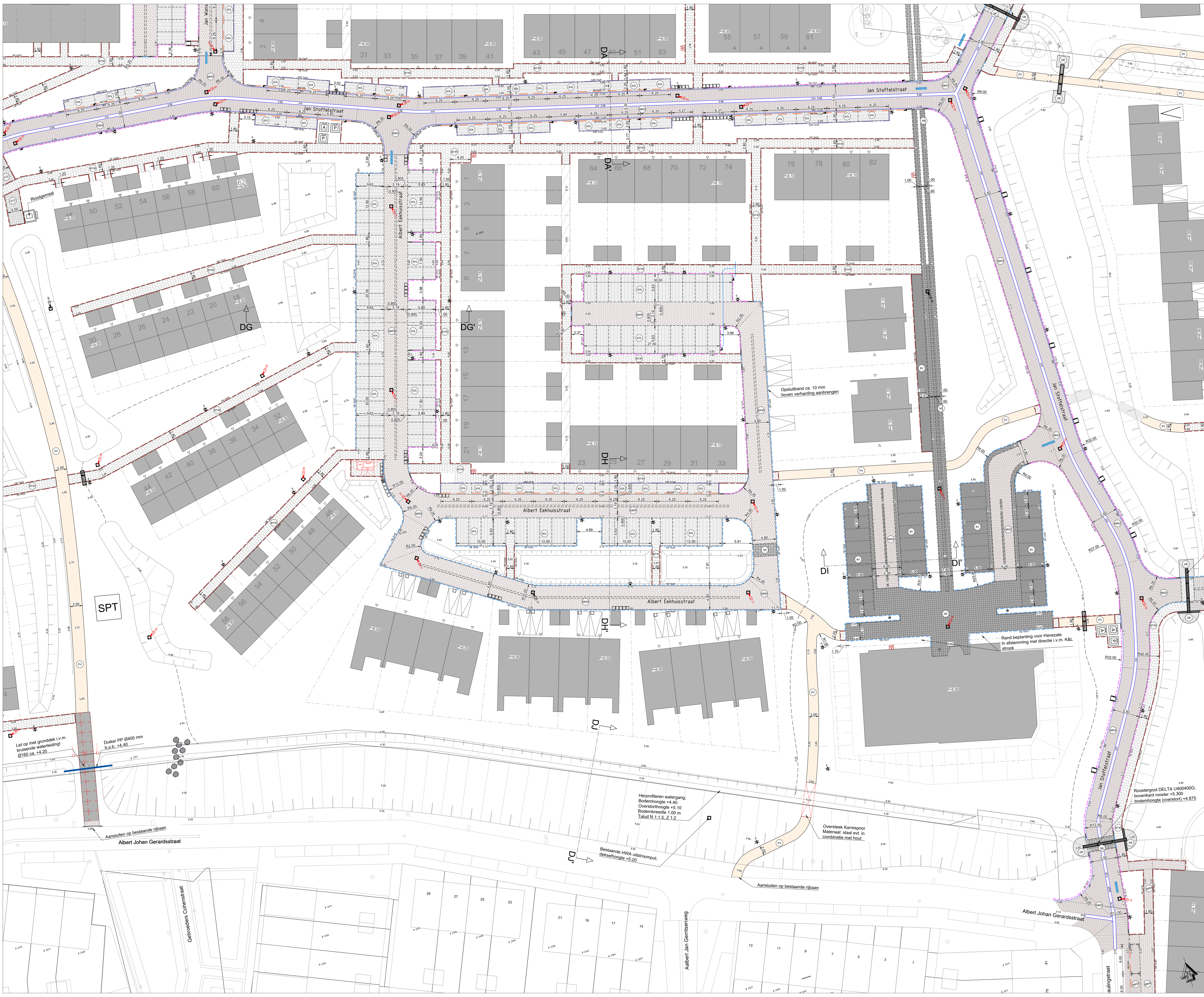
Overzichtstekening 1:5000
